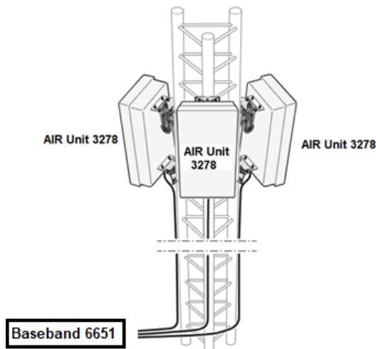
Slika 1. Blok šema povezivanja NR3600 RU jedinica sa baseband jedinicom
