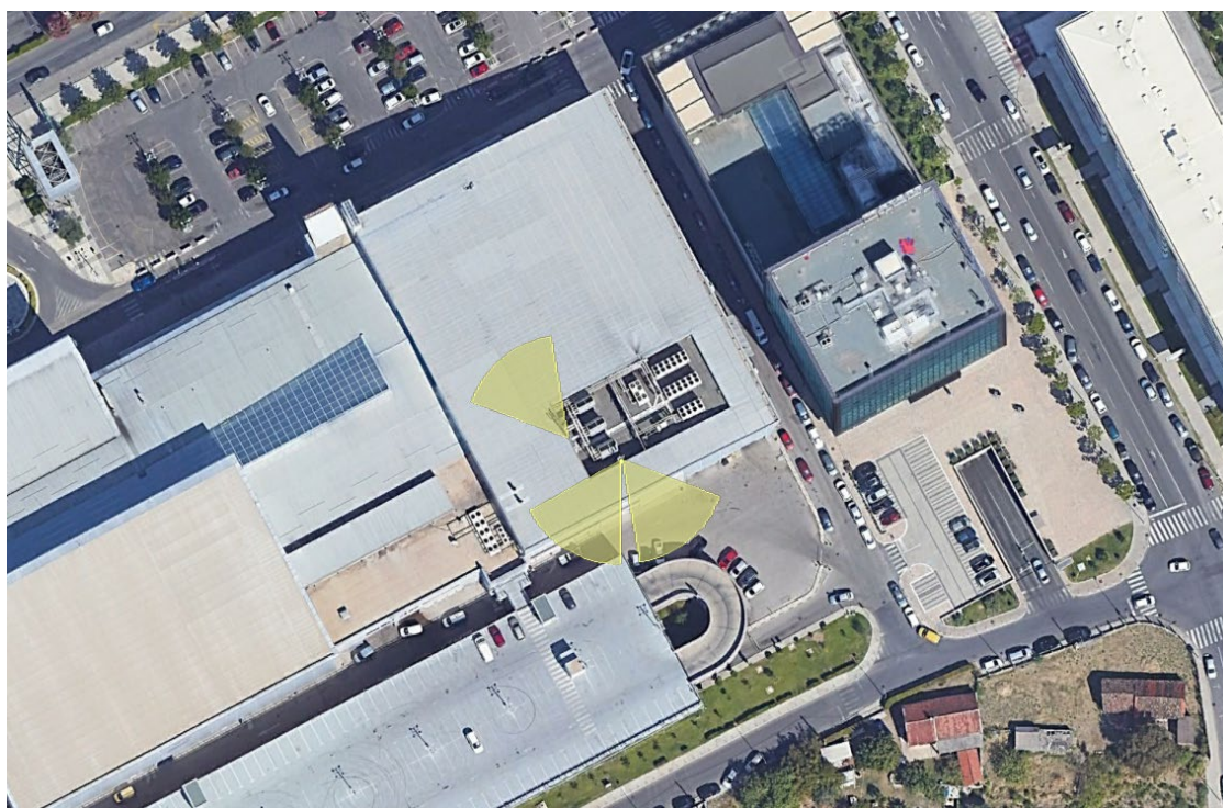
Slika 5. Pozicija antenskih nosača sa prikazanim azimutima Mtel antena, sa graničnom zonom i okolnim objektima
