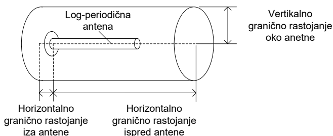
Slika 7.3. Zona nedozvoljenog zračenja za log-periodičnu antenu
