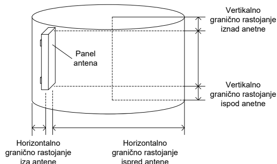
Slika 7.1. Zona nedozvoljenog zračenja za sektorsku panel antenu
