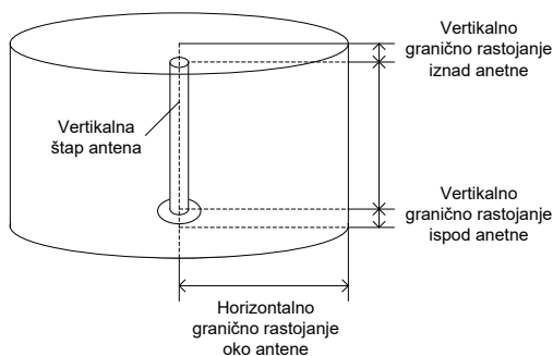
Slika 7.2. Zona nedozvoljenog zračenja za omnidirektivnu antenu
