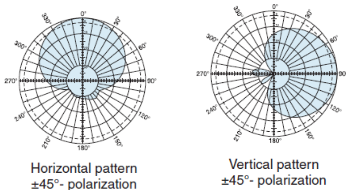
Dijagram zračenja antene K739 619
