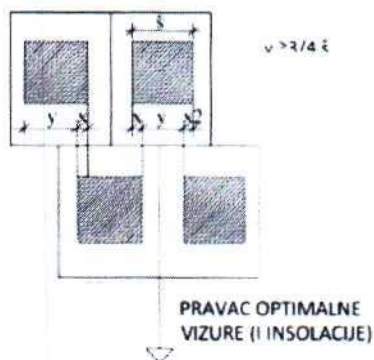
Slika 65: Uslovi za horizontalno postavljanje objekata na nagutim terenima
