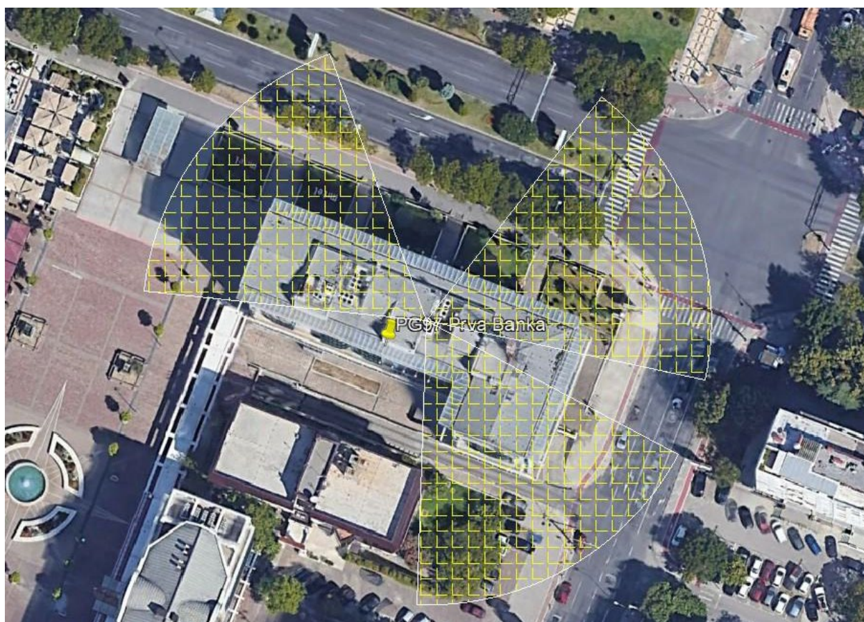
Slika 4.1 Pozicija antenskih nosača na objektu sa prikazanim azimutima antena, graničnom zonom i okolnim objektima
