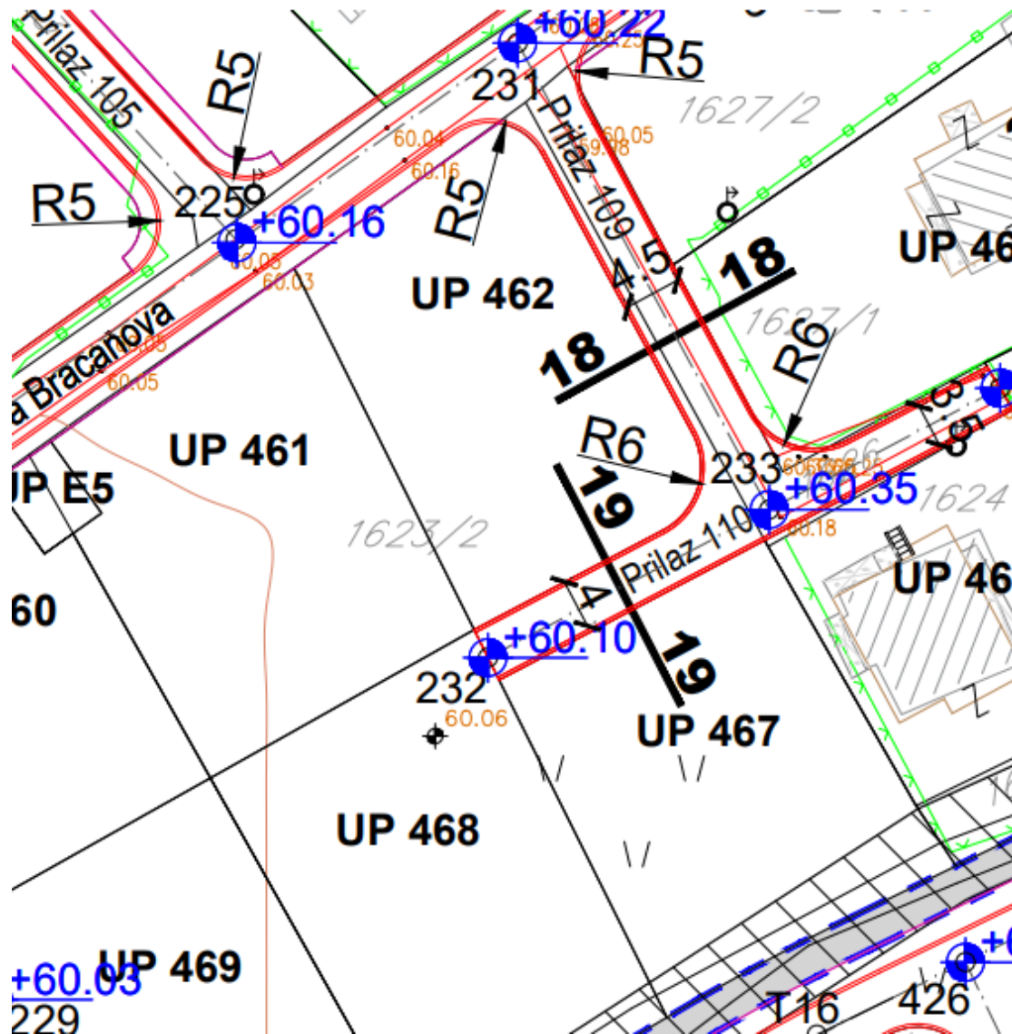
presjek 18-18
