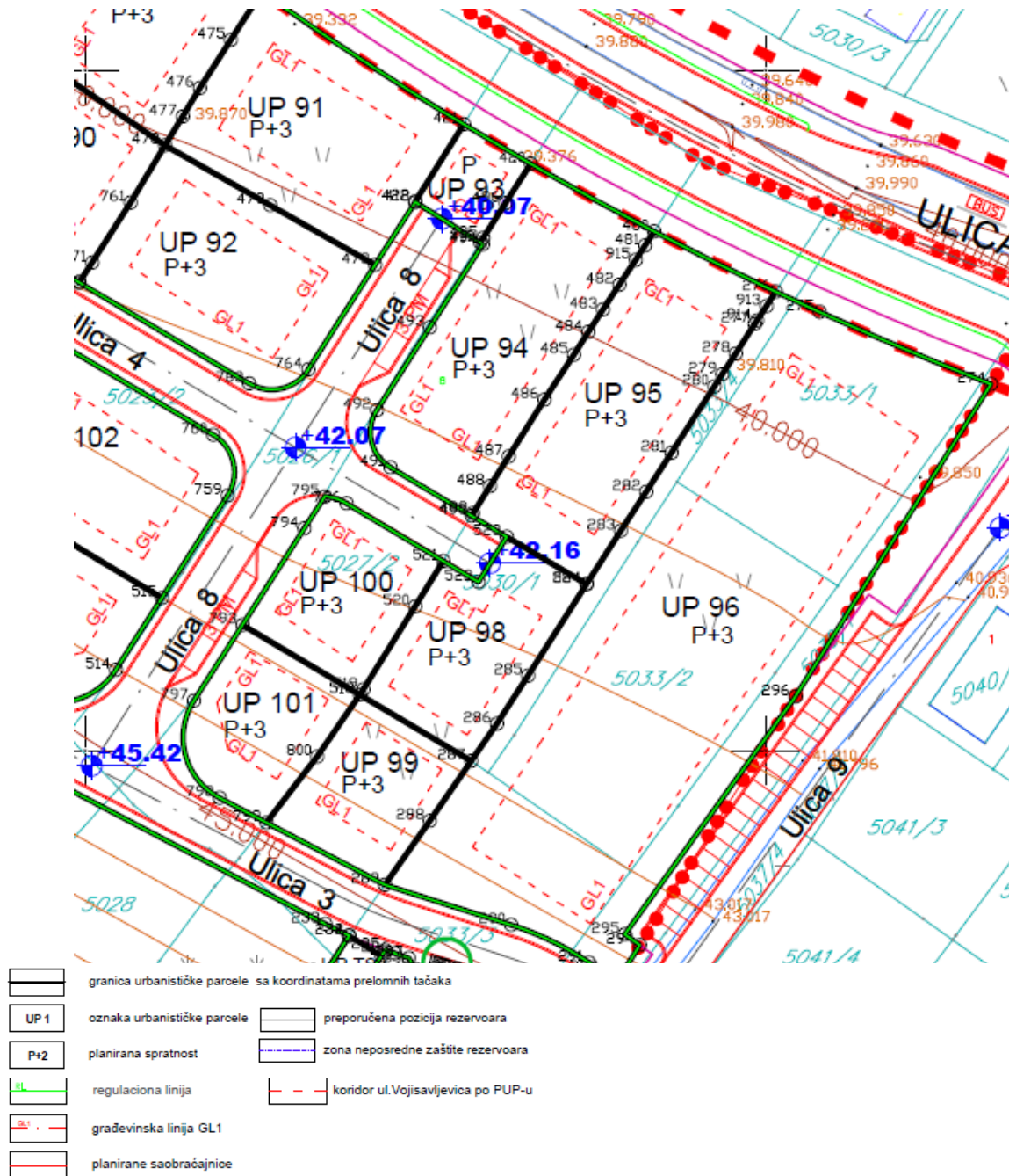
GRAFIČKI PRILOG – Plan parcelacija , regulacija i nivelacija sa koordinatama UP
