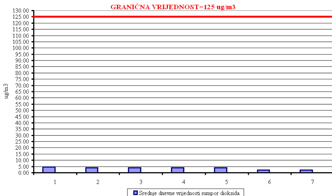
Slika 39. Srednje dnevne vrijednosti sumpor dioksida
