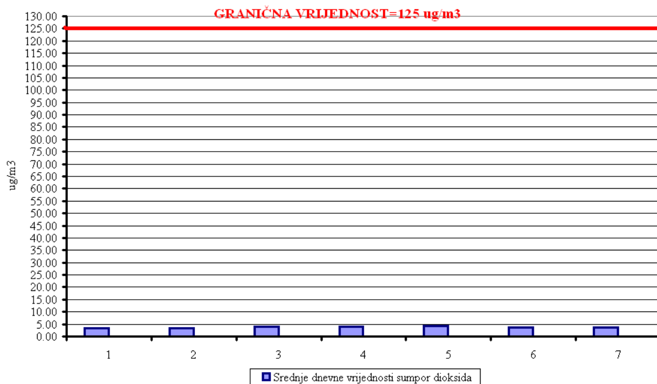
Slika 29. Srednje dnevne vrijednosti sumpor dioksid
