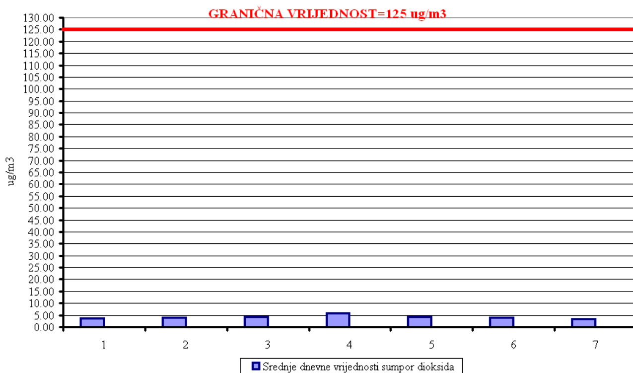
Slika 17. Srednje dnevne vrijednosti sumpor dioksida
