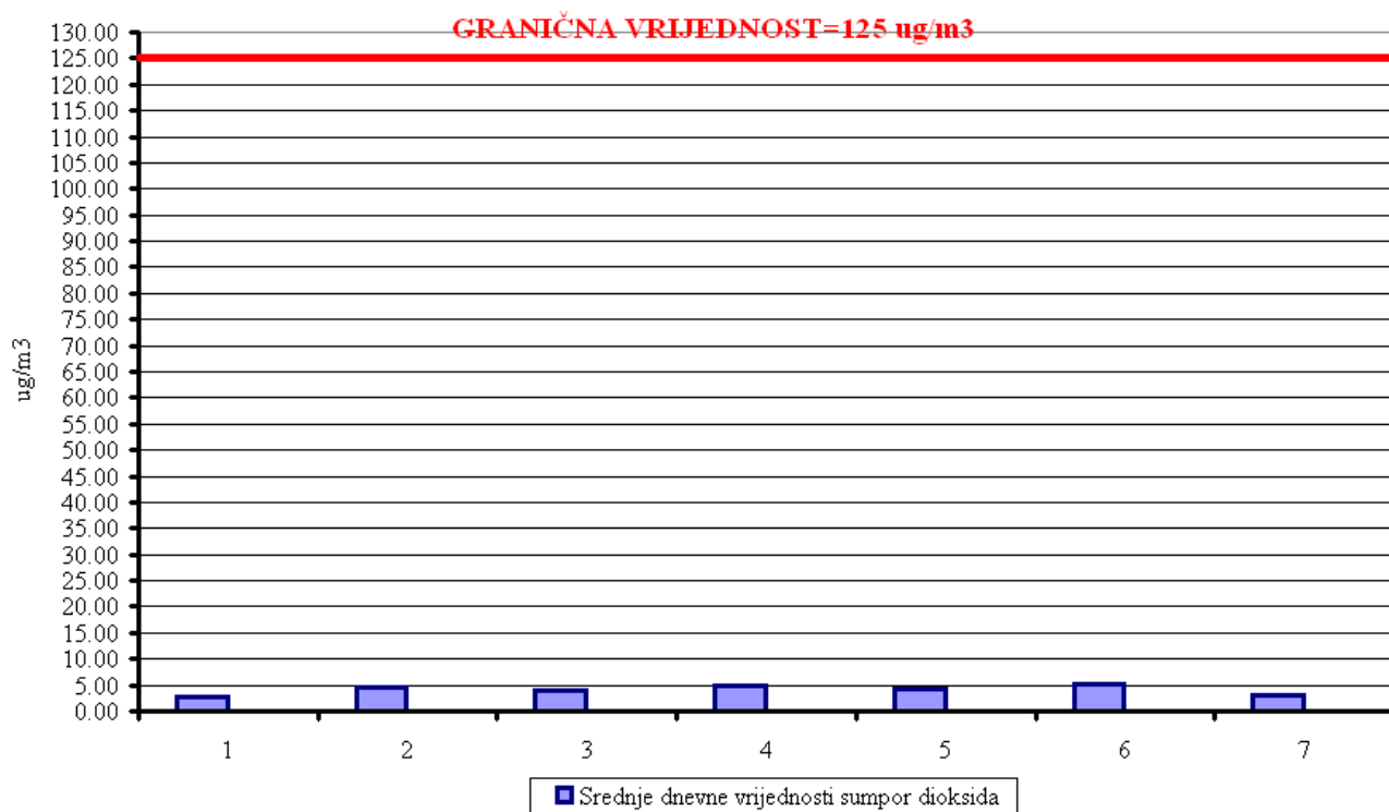
Slika 35. Srednje dnevne vrijednosti sumpor dioksida
