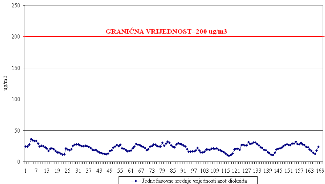
Slika 33. Jednočasovne srednje vrijednosti azot dioksida
